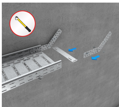
23 | Łuk pionowy wykonany z łączników (RGV)
