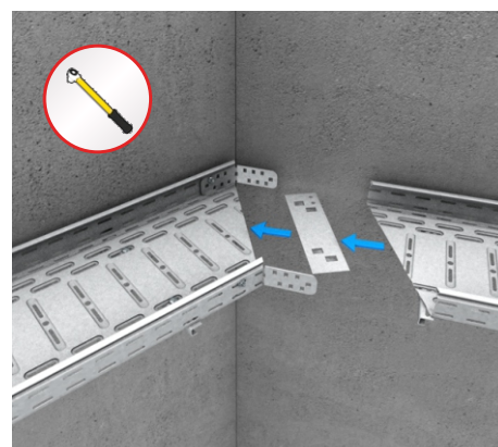
21 | Wykonanie zakrętu poziomego
