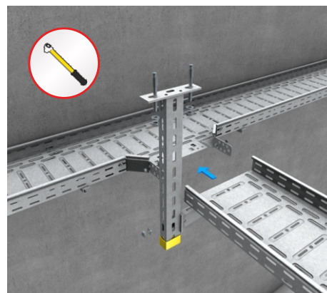
18 | Montaż korytka do elementu (RAE)
