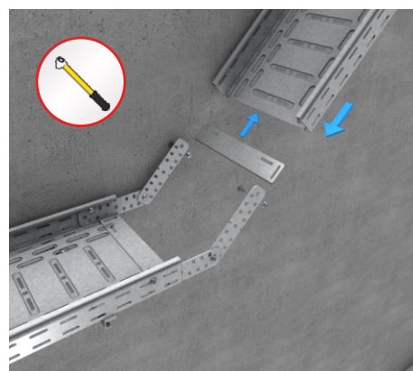
24 | Łuk pionowy wykonany z łączników (RGV)
