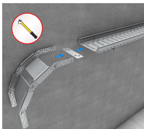
22 | Łuk pionowy korytka kablowego (RVB)
