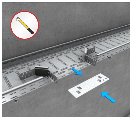
17 | Montaż rogowego elementu do dobudowania (RAE)
