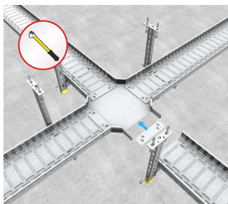
19 | Skrzyżowanie korytek (RK)
